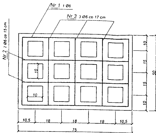
e) Płyta 0,75 \times 0,50 \times 0,07 m z otworami kwadratowymi
