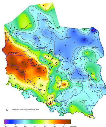
Rysunek 15 Mapa rozkładu gęstości ziemskiego strumienia ciepłego na obszarze Polski Źródło: Szewczyk J., Giętka D., 2009, [za:] Wójcicki A., Sowizdżał A., Bujakowski W., 2013
