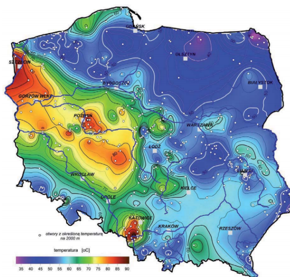
Rysunek 16 Mapa rozkładu temperatury na głębokości 2 km Źródło: Szewczyk J., 2010, [za:] Wójcicki A., Sowizdżał A., Bujakowski W., 2013
