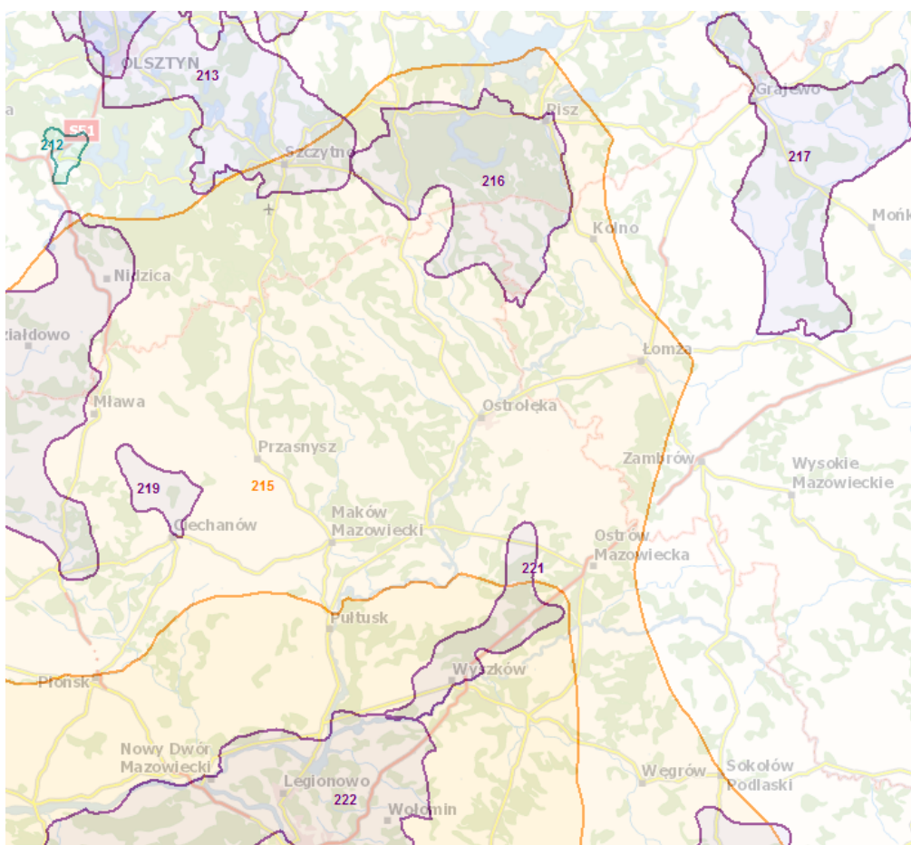
Rysunek 19 Główne Zbiorniki Wód Podziemnych w rejonie miasta Ostrołęka
