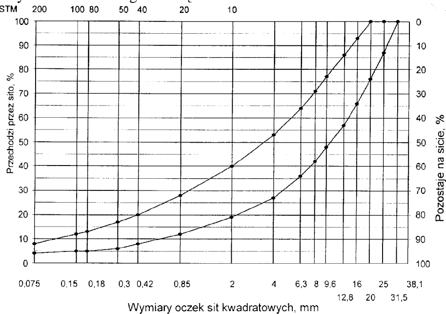
Rys. 2. Krzywe graniczne uziarnienia mieszanki mineralnej BA od 0 do 25mm do podbudowy nawierzchni drogi o obciążeniu ruchem KR 1 lub KR 2
