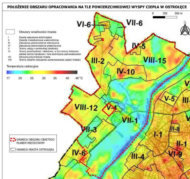
Rysunek 16 Położenie obszaru opracowania na tle powierzchniowej wyspy ciepła ( Strategia adaptacji miasta Ostrołęki do zmian klimatu do roku 2025 z perspektywą do 2030 (projekt) )
