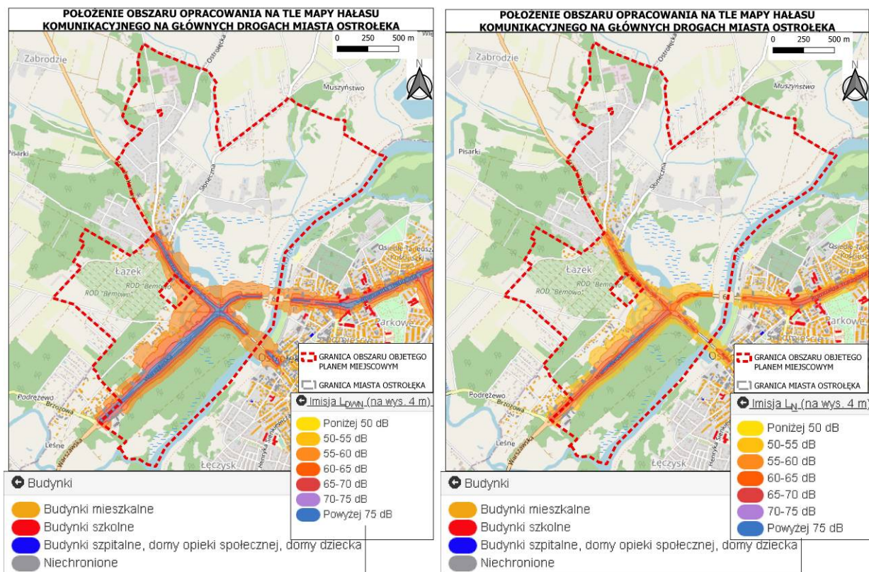
Rysunek 19 Mapa obrazująca stan akustyczny środowiska wyrażony wskaźnikami LDWN i LN w postaci barwnych stref, ilustrujących przedziały zakresu emisji ( http://mapy-akustyczne.bip.um.ostroleka.pl/ )
