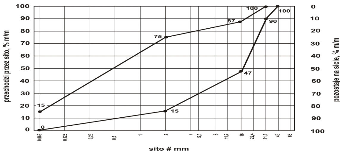
Rys. 1. Uziarnienie mieszanki niezwiązanej 0/31,5 do warstwy odsączającej
