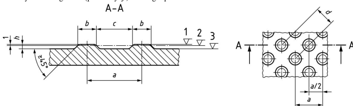
Rys. 1a. Płytki ostrzegawcza (pole decyzji) – szczegół powierzchni
