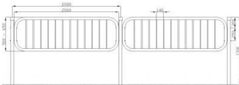
Przykład ogrodzenia typu „olsztyńskiego” z wypełnienia rysunek poglądowy
