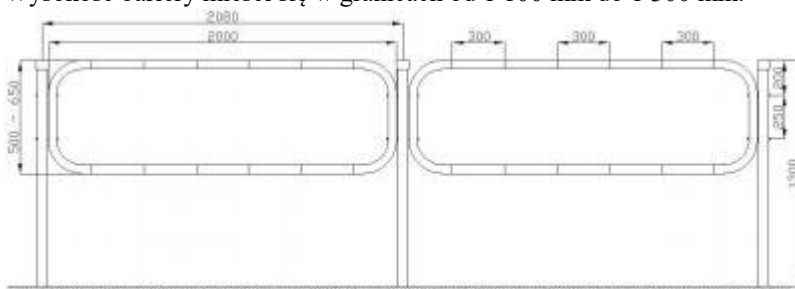
Przykład ogrodzenia typu „olsztyńskiego” bez wypełnienia rysunek poglądowy
