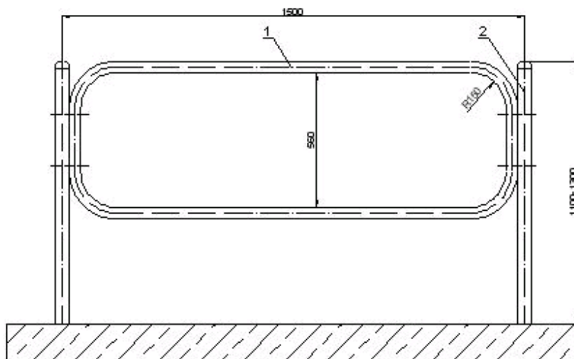
Rys. 1. Wzór bariery ochronnej z rur stalowych (typ „olsztyński”)
