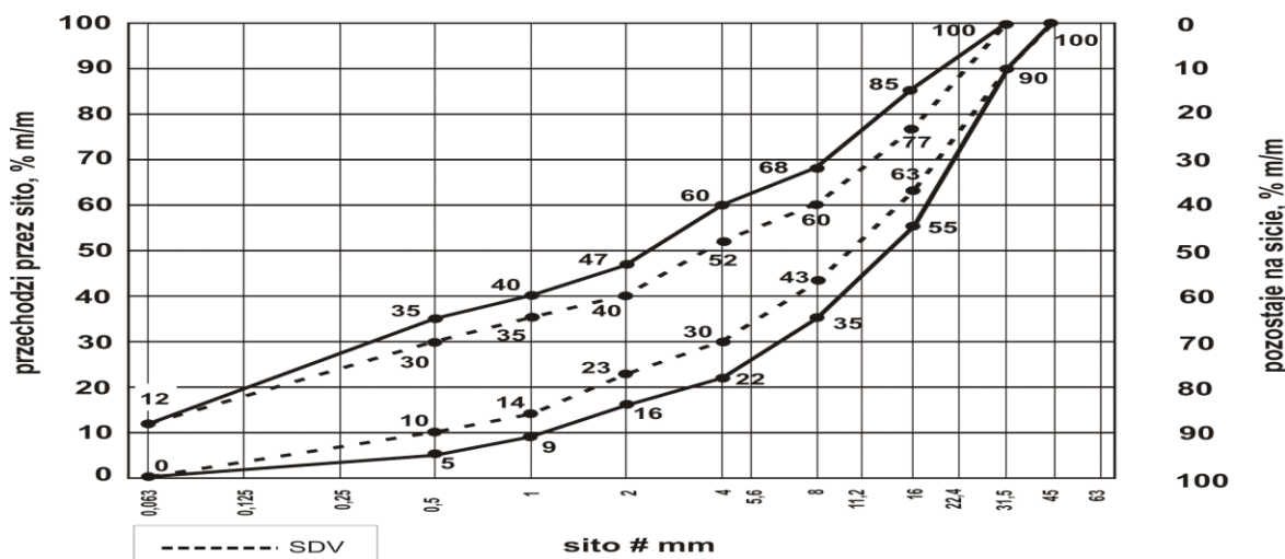
Rys. 2. Uziarnienie mieszanki niezwiązanej 0/31,5 dla podbudowy pomocniczej poszerzenia zjazdu publicznego
