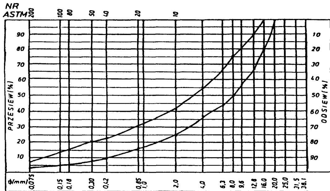
Rys. 12. Krzywe graniczne uziarnienia mieszanki mineralnej 0,20 mm do warstwy wiążącej, wyrównawczej i wzmacniającej z betonu asfaltowego dla KR 3-6
