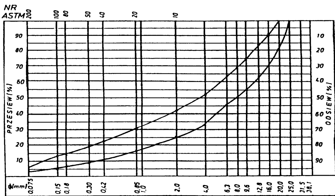
Rys. 11. Krzywe graniczne uziarnienia mieszanki mineralnej 0,25 mm do warstwy wiążącej, wyrównawczej i wzmacniającej z betonu asfaltowego dla KR 3-6
