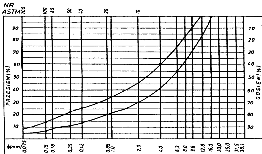
Rys. 13. Krzywe graniczne uziarnienia mieszanki mineralnej 0,16 mm do warstwy wiążącej, wyrównawczej i wzmacniającej z betonu asfaltowego dla KR 3-6
