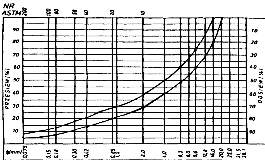
Rys. 4. Krzywe graniczne uziarnienia mieszanki mineralnej 0,20 mm do warstwy ścieralnej z betonu asfaltowego dla KR 3-6
