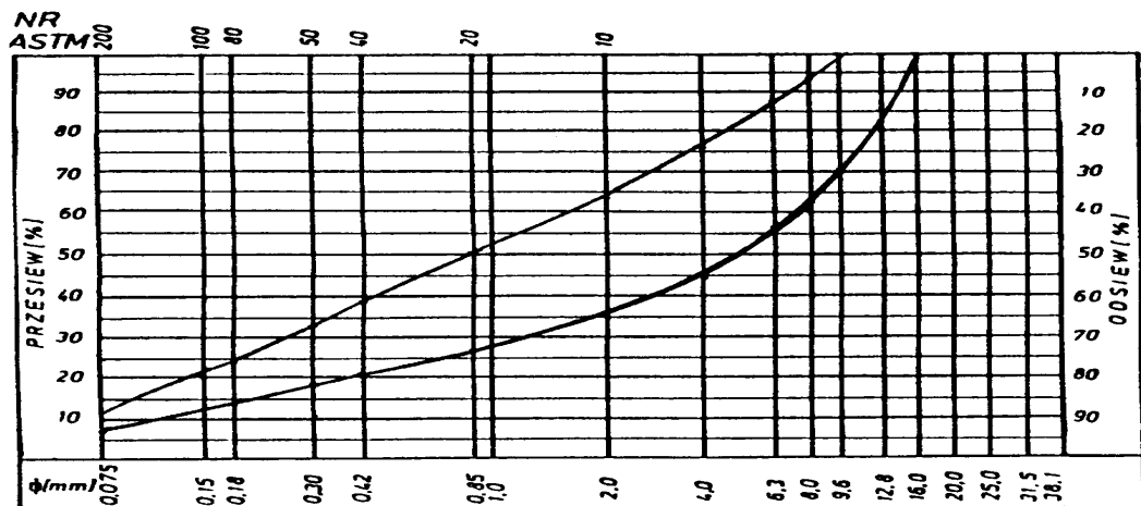
Rys. 2. Krzywe graniczne uziarnienia mieszanki mineralnej 0,16, 0,12,8 mm do warstwy ścieralnej z betonu asfaltowego dla KR 1-2
