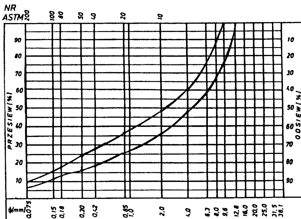
Rys. 7. Krzywe graniczne uziarnienia mieszanki mineralnej 0,12,8 mm do warstwy ścieralnej z betonu asfaltowego dla KR 3-6
