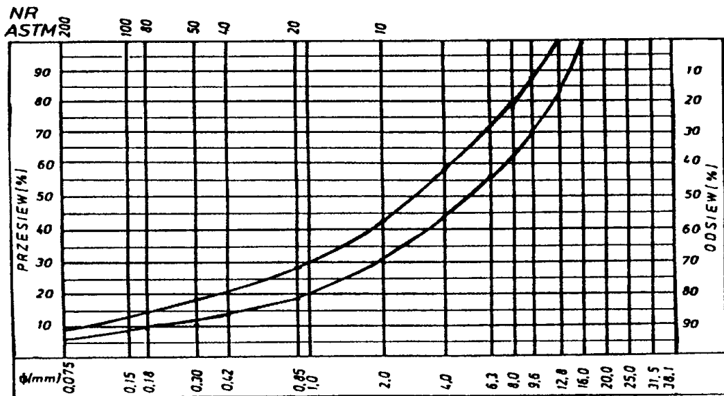
Rys. 6. Krzywe graniczne uziarnienia mieszanki mineralnej 0,16 mm do warstwy ścieralnej z betonu asfaltowego dla KR 3-6
